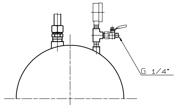
A矢視図
